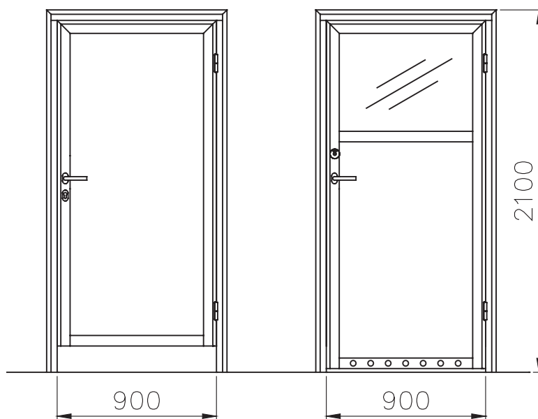
rysunek schematyczny
