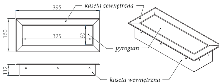
rysunek schematyczny
