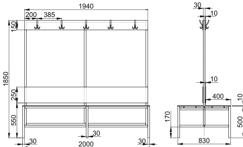
rysunek schematyczny
