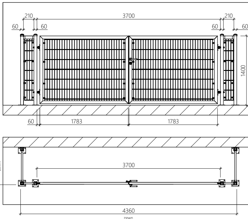
rysunek schematyczny
