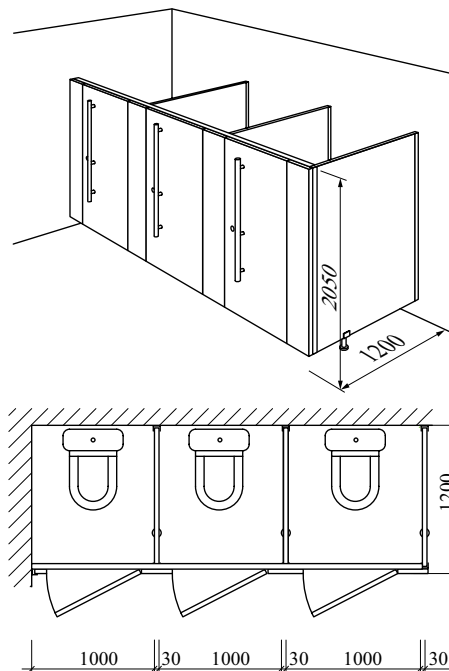
rysunek schematyczny
