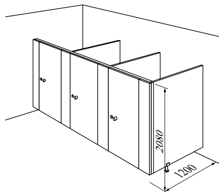
rysunek schematyczny
